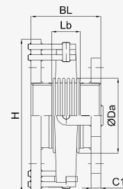
DN 100 - DN 700
