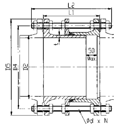
ТАБЛИЦЯ РОЗМІРІВ ДЛЯ ТИСКУ PN25
